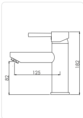
Смеситель для раковины, картридж 35мм Sedal, аэратор Neoperl, гибкая подводка
